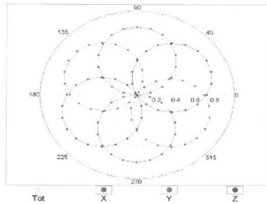
f=1800 MHz,R22
