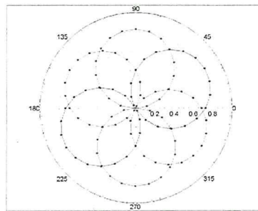
f=1800 MHz,R22
