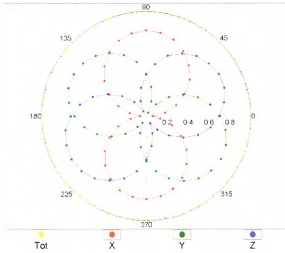
f=450 MHz,TEM
