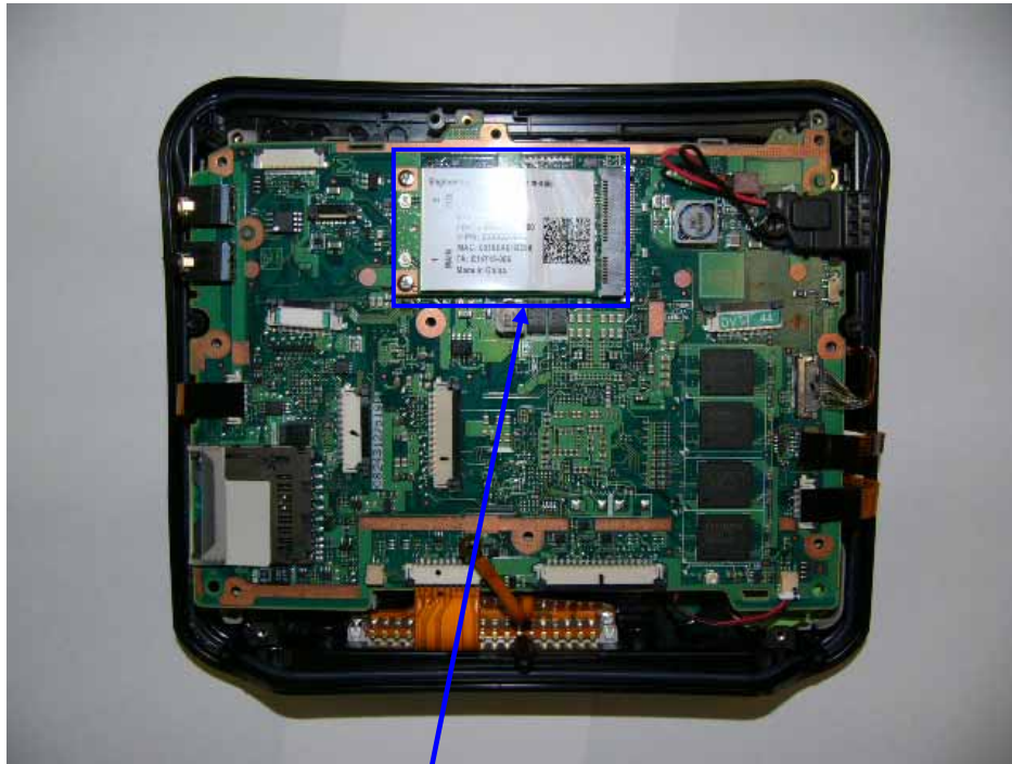
WLAN Module
