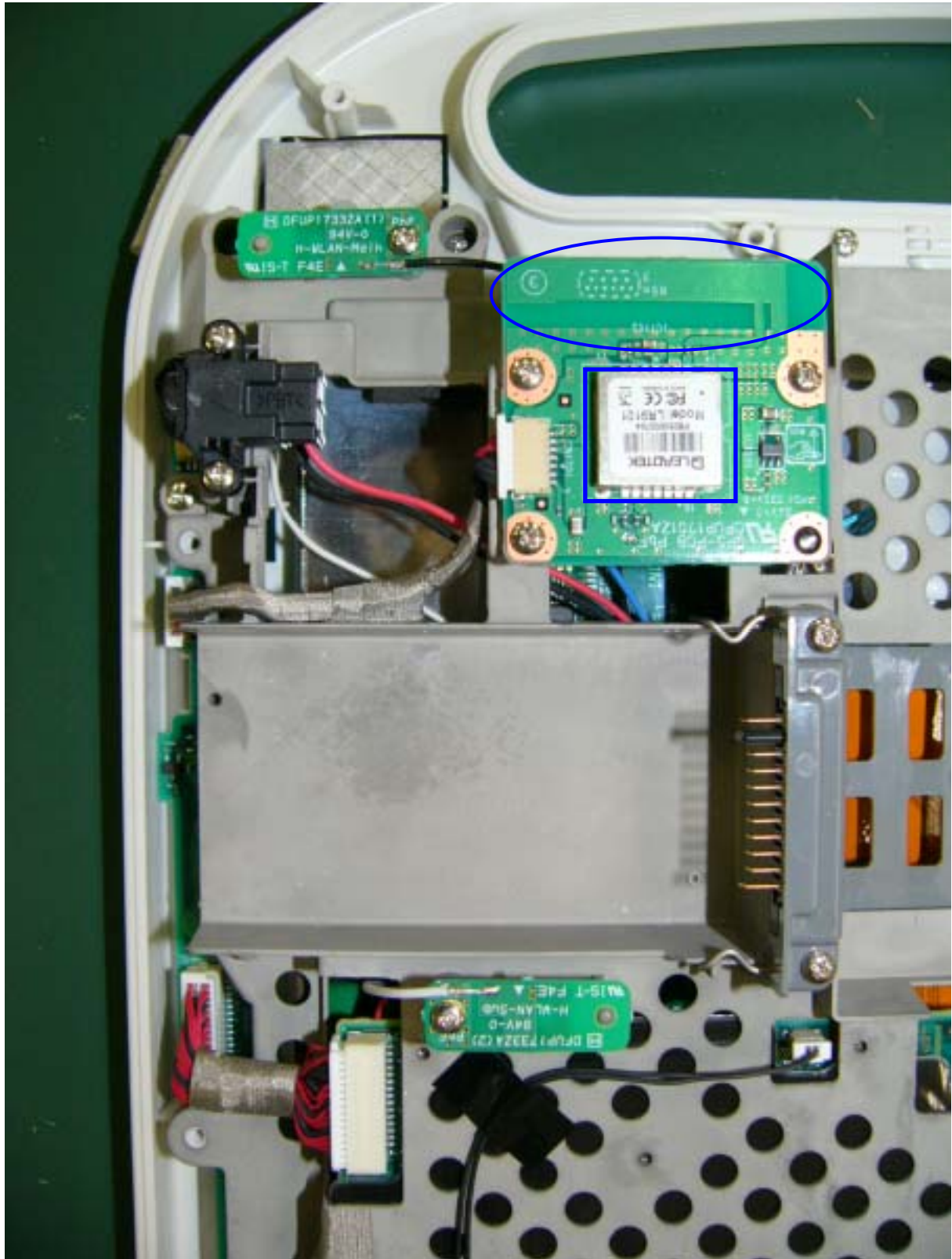
GPS Module & RX Antenna
