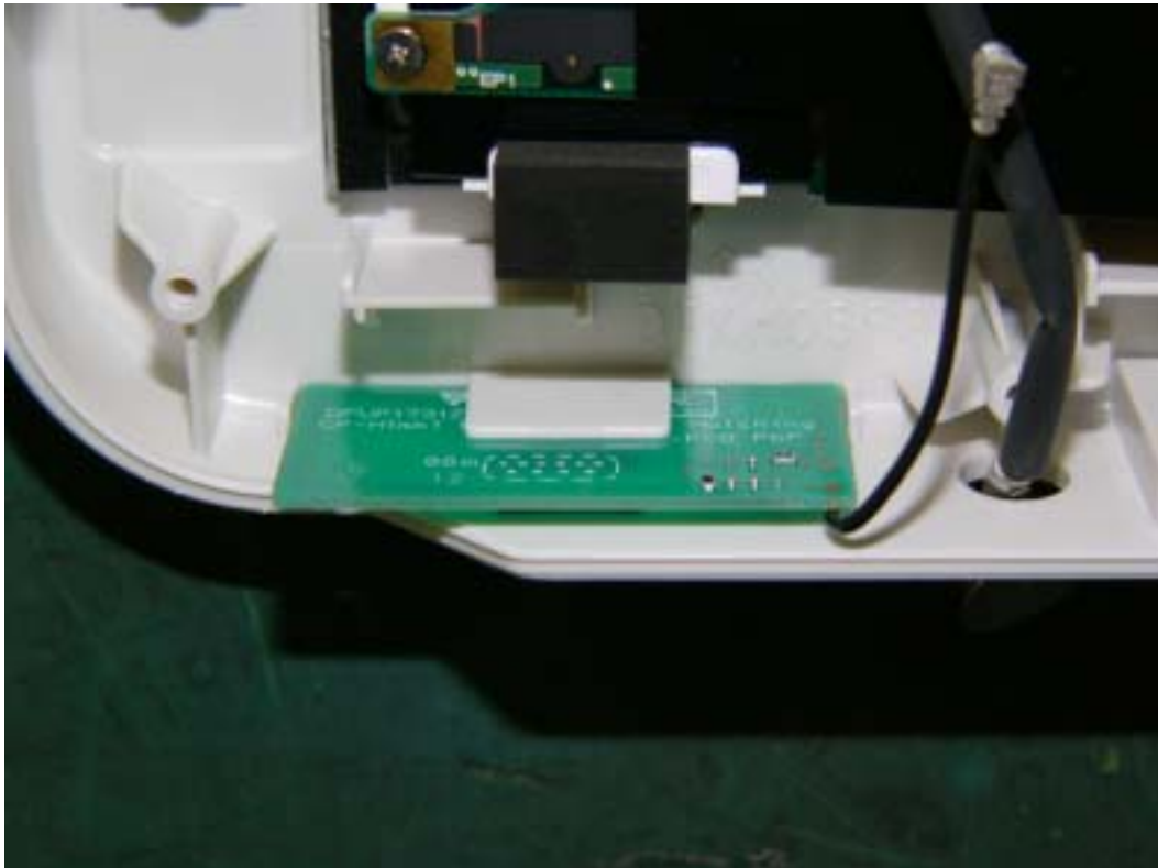
RFID TX/RX Antenna
