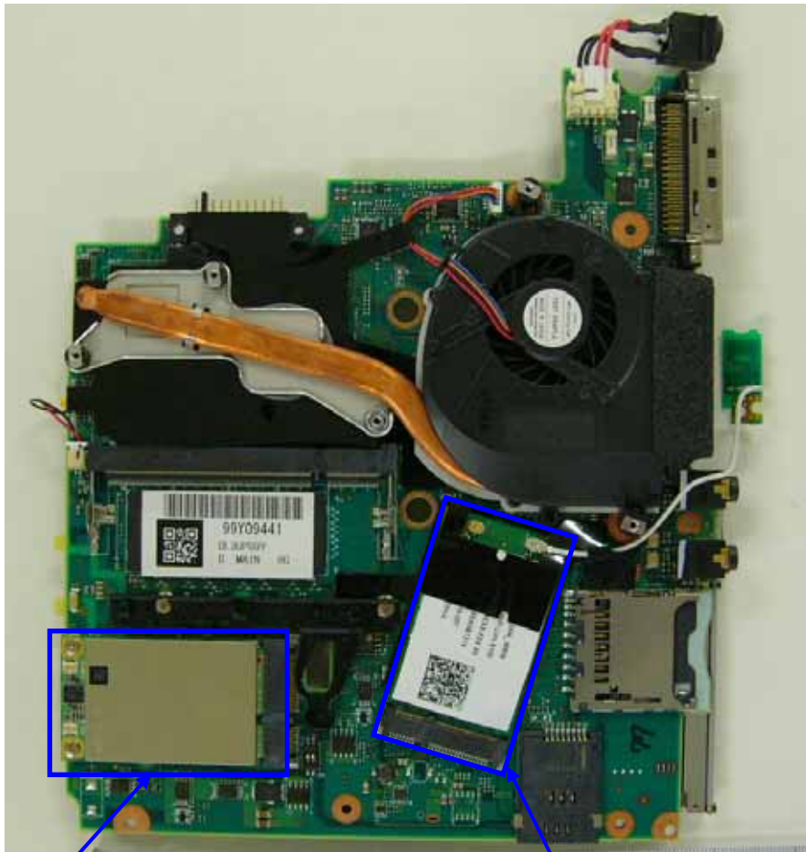
WWAN Module
