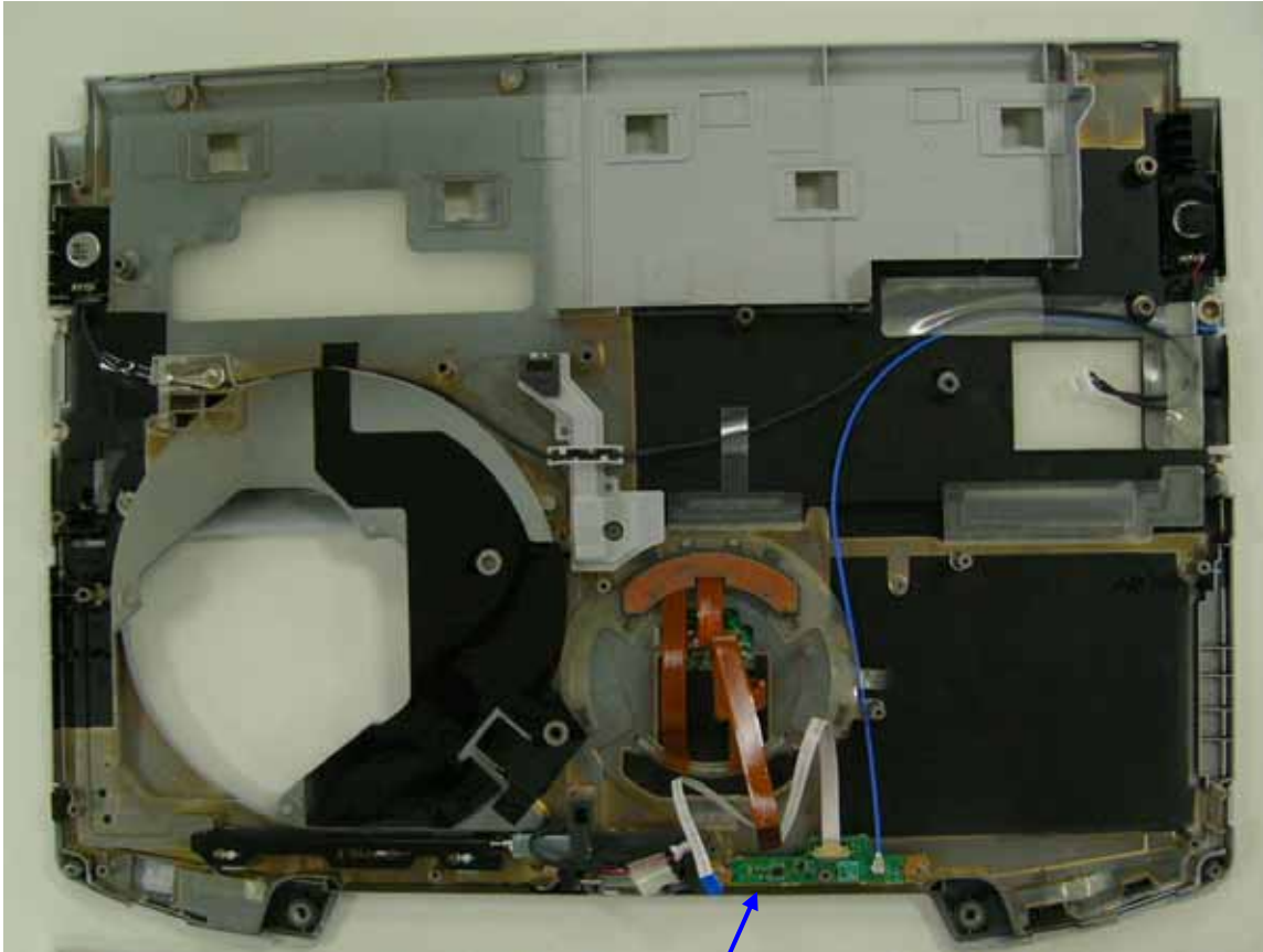
Bluetooth Module
