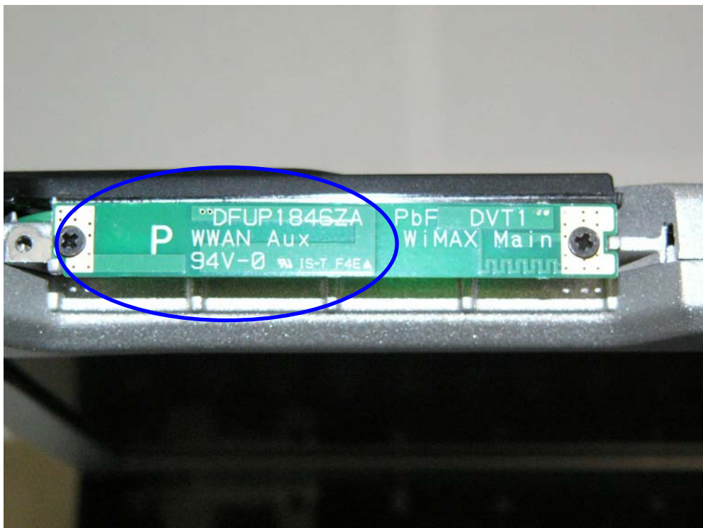
WWAN Aux /GPS(Gobi2000) RX Antenna
