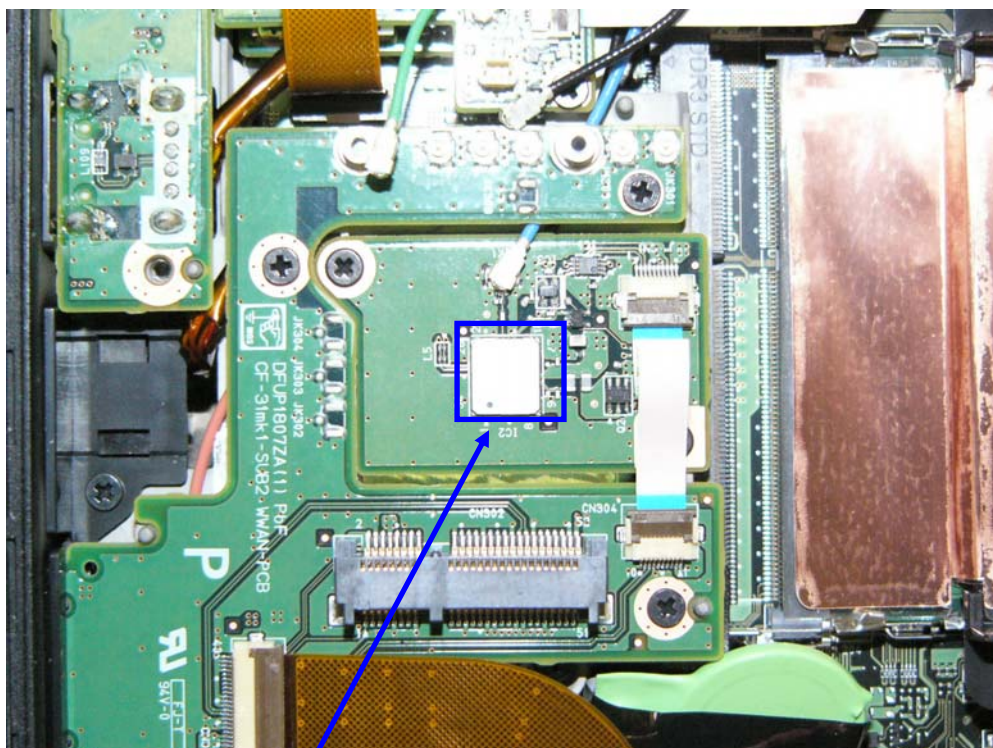
Bluetooth Module
