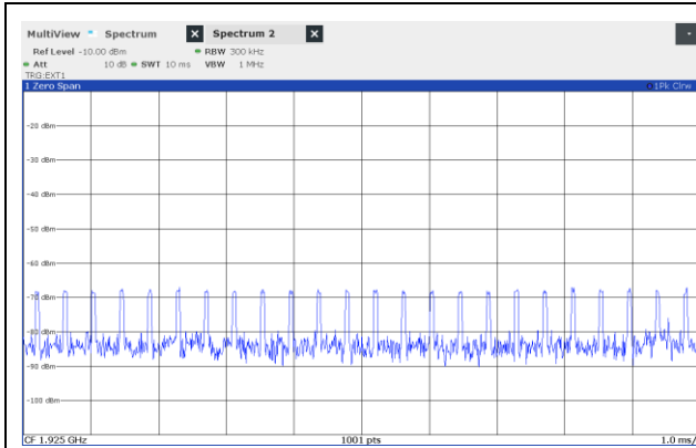
50 µs Pulses
