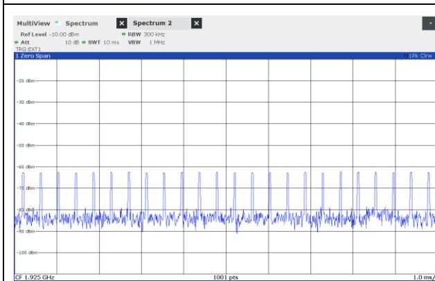
35 µs Pulses
