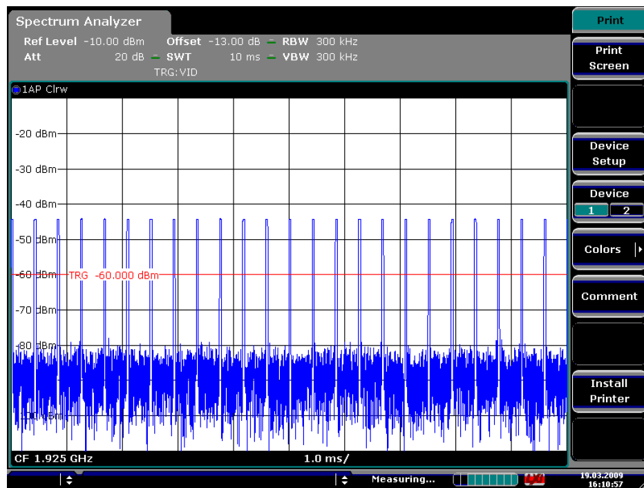
35 µs Pulses
