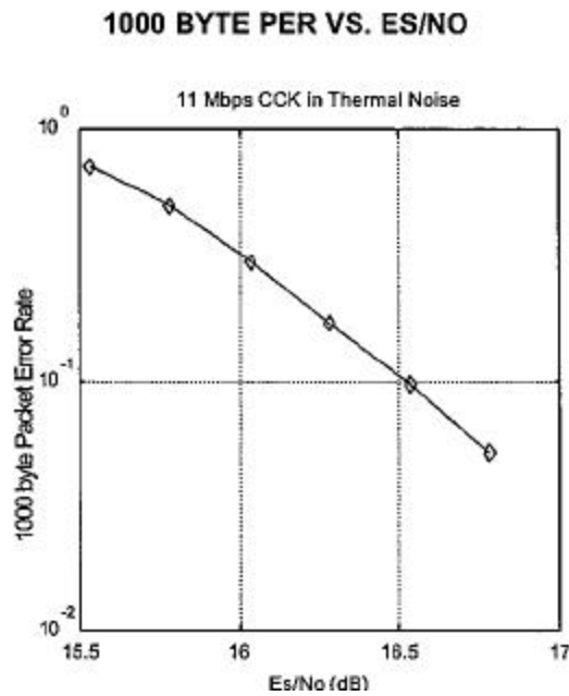
figure.1 1000 byte PER vs. Es/No
