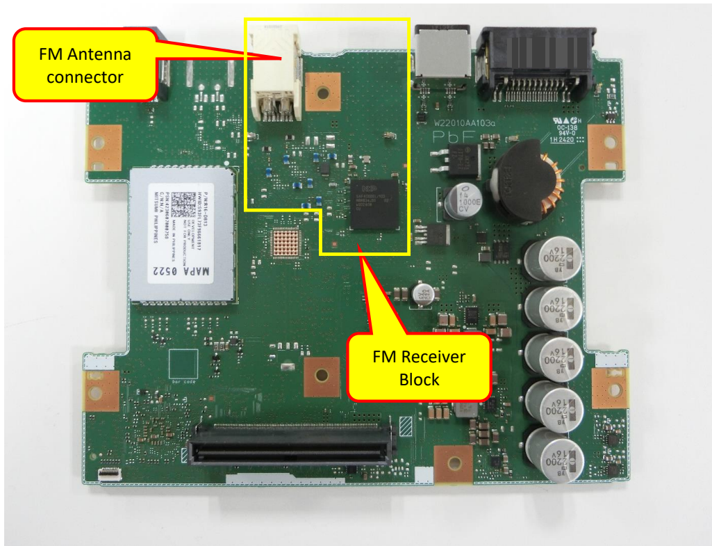
【Figure 5】 AUDIO_PCB (Surface Side)
