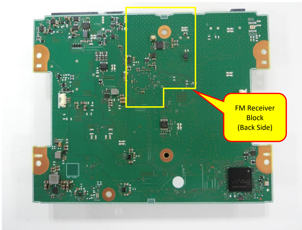
【Figure 6】 AUDIO_PCB (Back Side)
