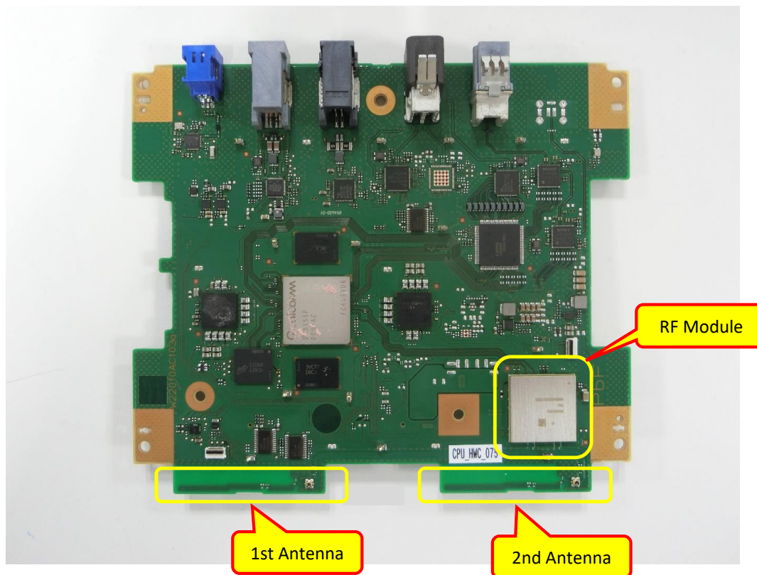
【Figure 2】 CPU_PCB (Back Side)
