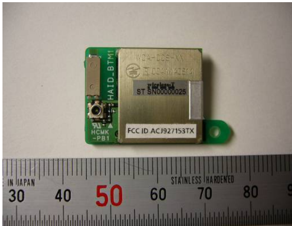
13) Bluetooth Module Top View
