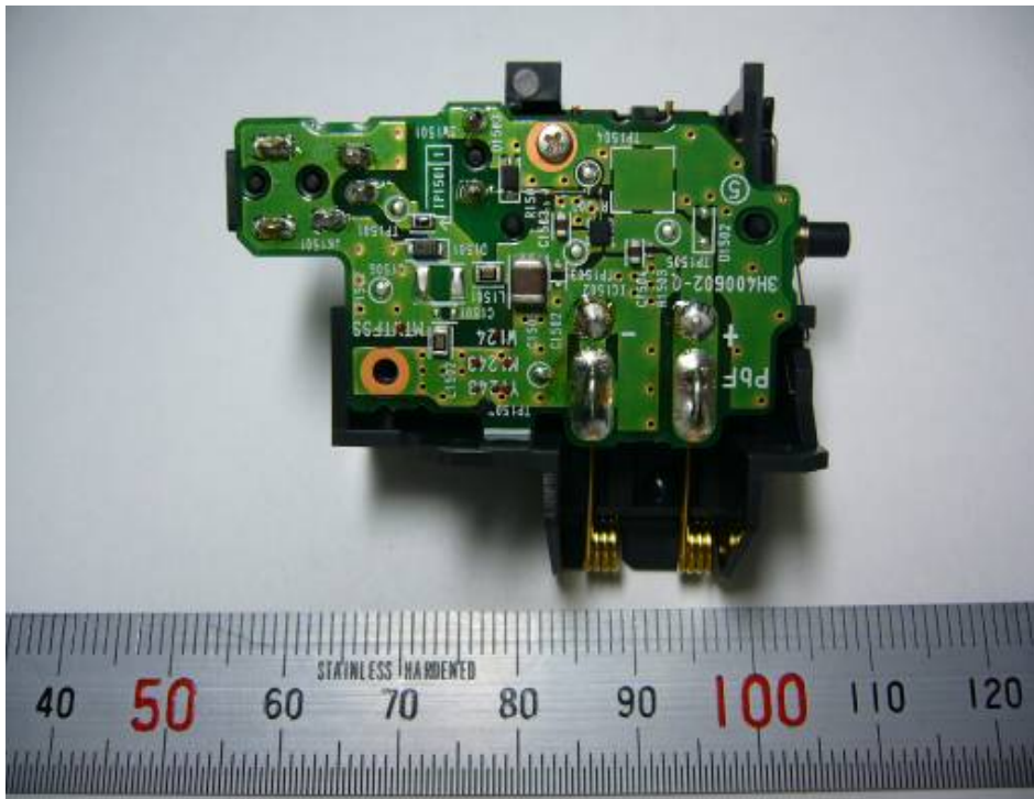
23) Chager cradle PCB View 1
