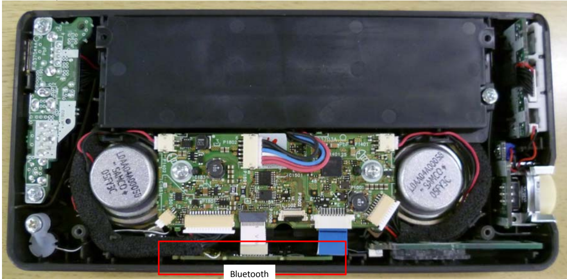
Bluetooth Module PCB
