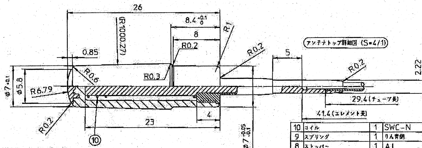
ホルダー詳細図 (S=4/1)
