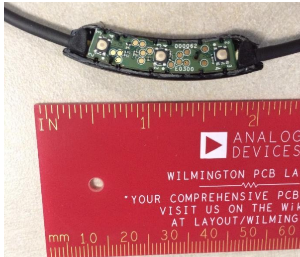
Button module
