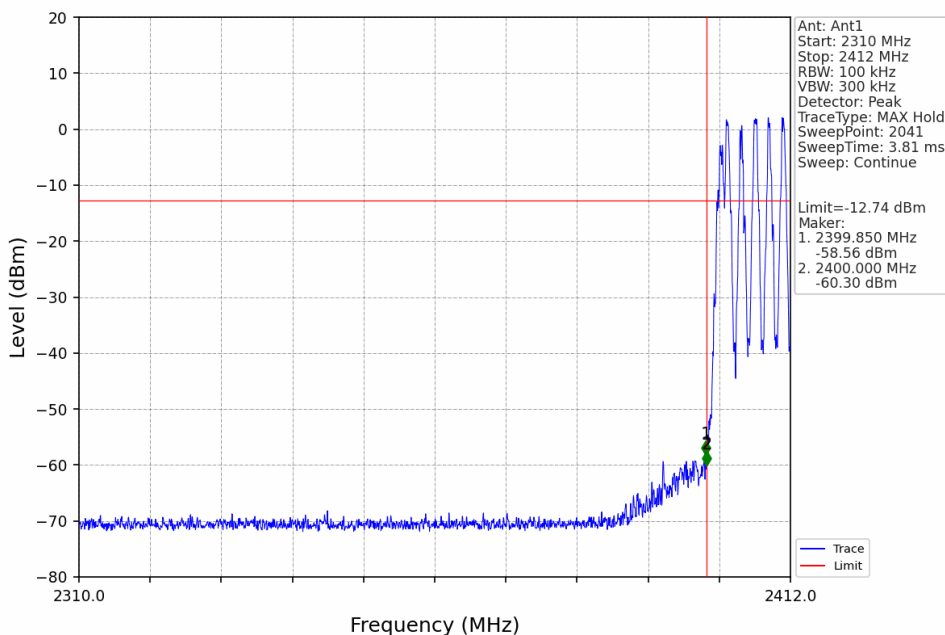
QHS6_HOPP_Ant1_NTNV
