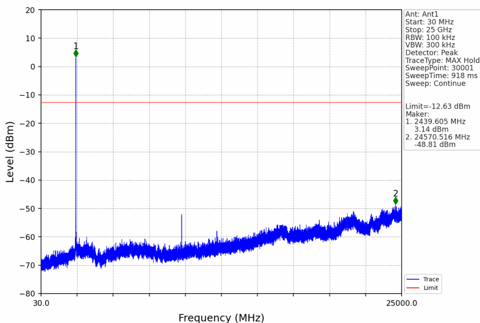
QHS2_MCH_2440MHz_Ant1_NTNV
