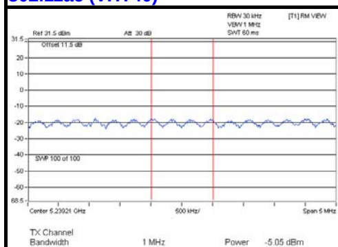
802.11ac (VHT40)
