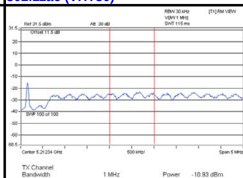
802.11ac (VHT80)
