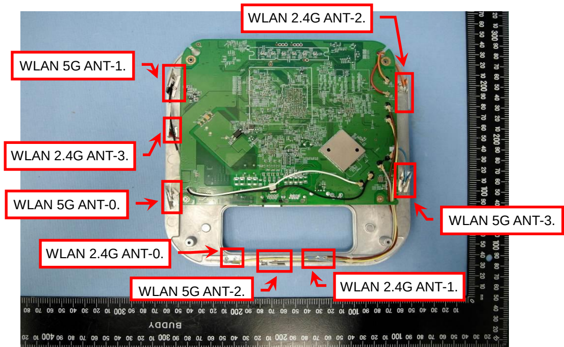
EUT Photo (2)
