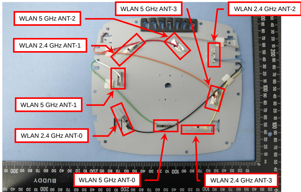
EUT Photo (18)
