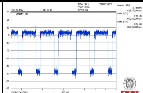
802.11n (40MHz)
