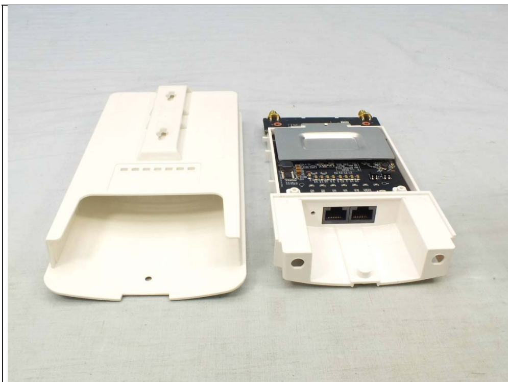
Model: ENS500EXT-AC
