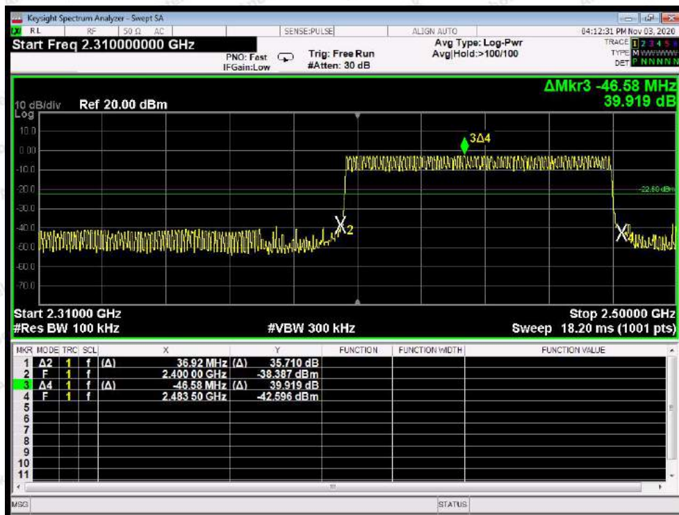
EDR mode- \pi/4 QPSK
