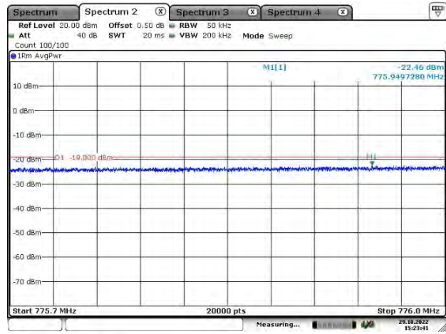
Left Side-WCDMA-Above AGC
