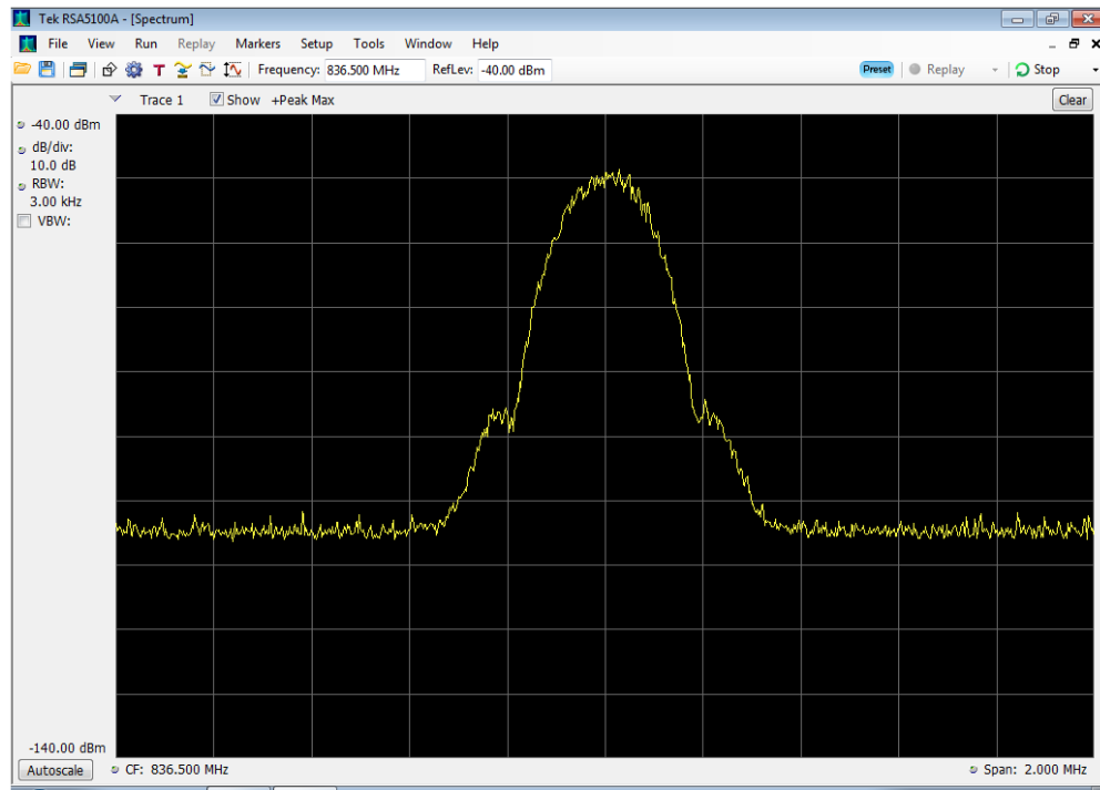
GSM Input_824-849MHz
