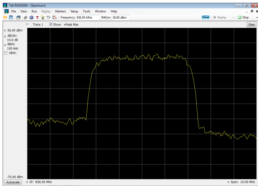
WCDMA output_824-849MHz
