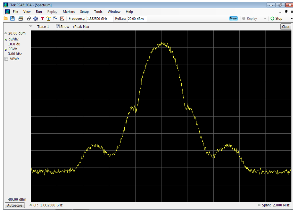
GSM output_1850-1915 MHz
