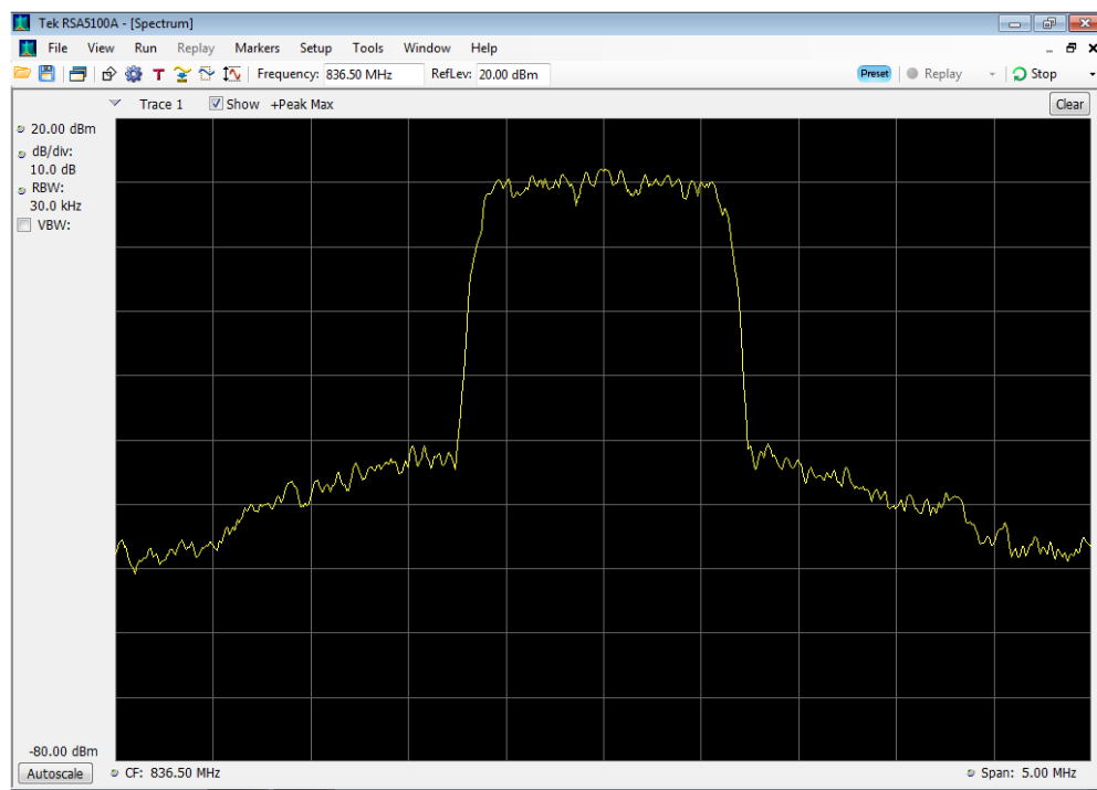
CDMA output_824-849MHz
