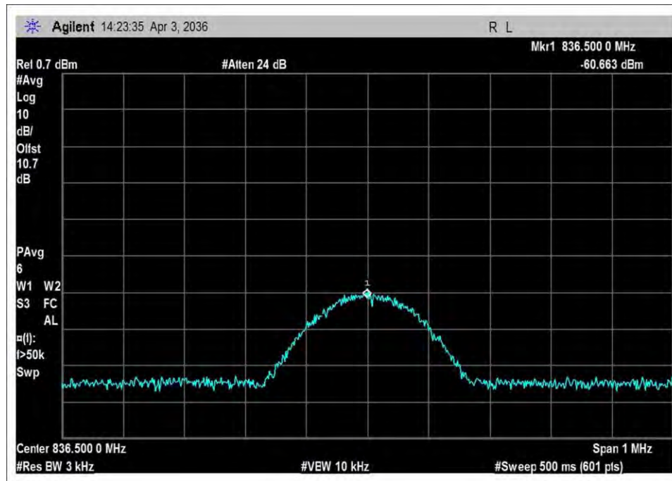
UL_824-849_input_GSM
