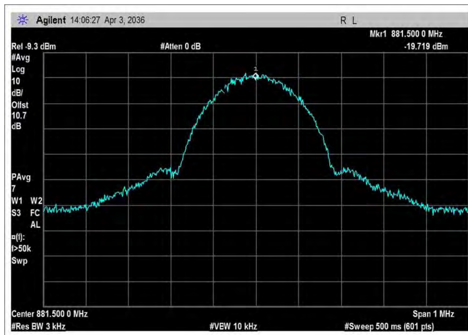
DL_869-894_output_GSM
