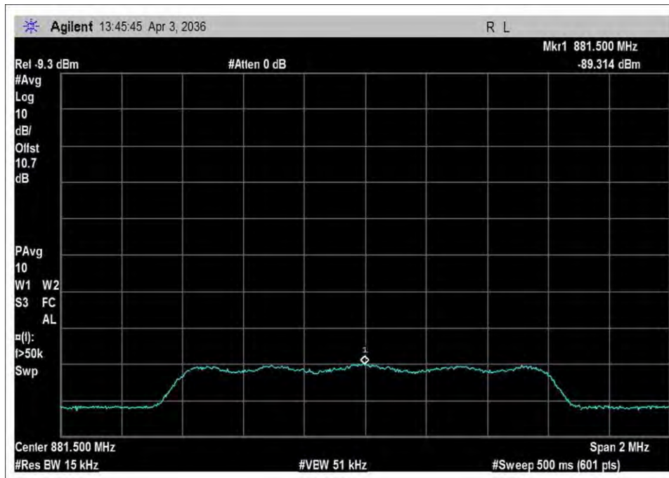
DL_869-894_input_CDMA
