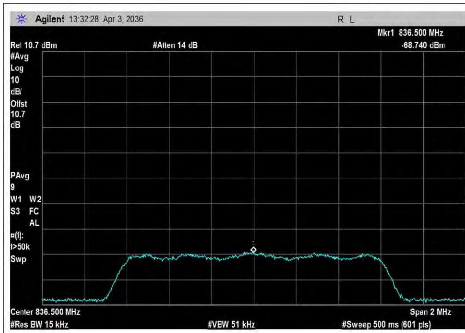
UL_824-849_input_CDMA
