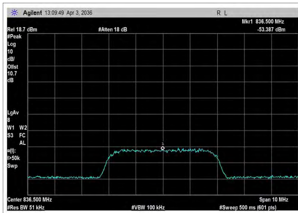
UL_824-849_input_WCDMA
