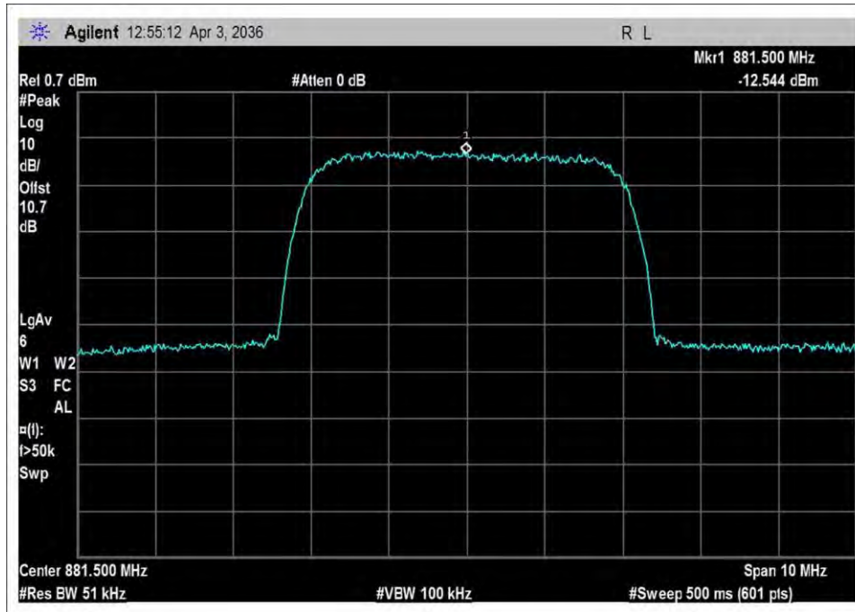
DL_869-894_input_WCDMA
