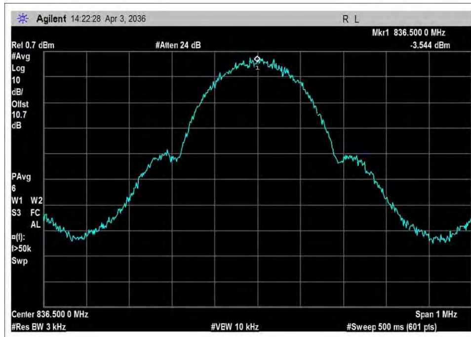
UL_824-849_output_GSM
