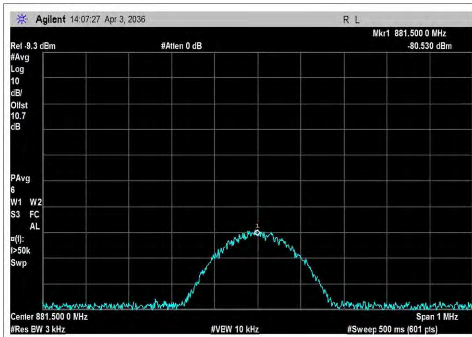
DL_869-894_input_GSM
