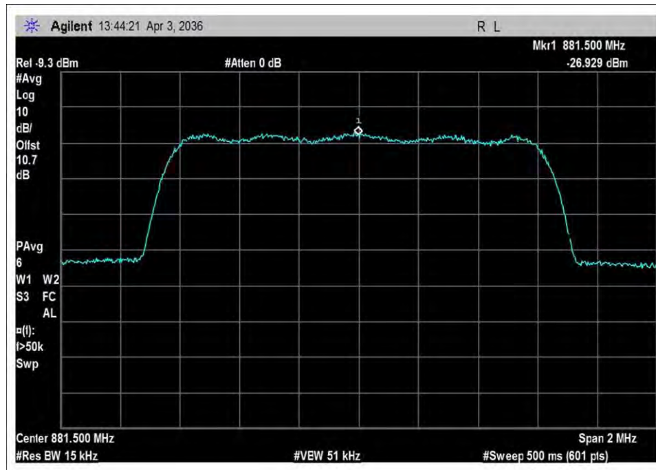
DL_869-894_output_CDMA
