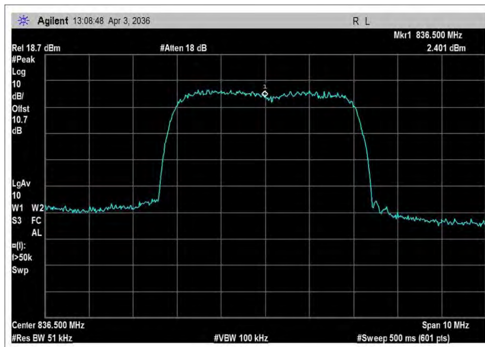
UL_824-849_output_WCDMA
