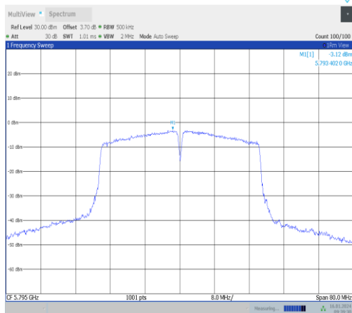
11n40ISO-Ant1-5795-PASS
