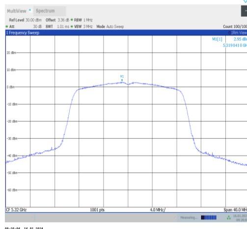
11n20ISO-Ant1-5320-PASS
