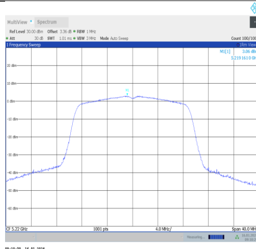
11n20ISO-Ant1-5220-PASS
