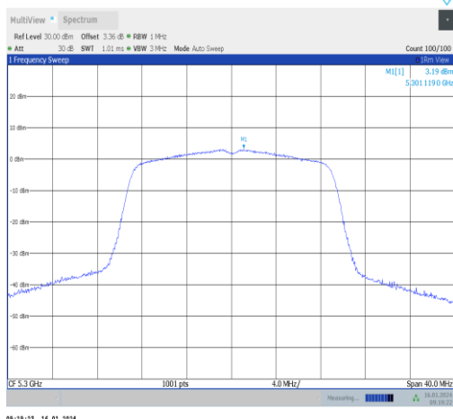
11n20ISO-Ant1-5300-PASS
