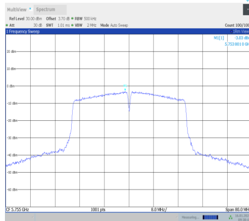
11n40ISO-Ant1-5755-PASS
