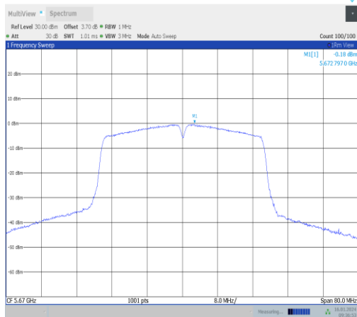
11n40ISO-Ant1-5670-PASS
