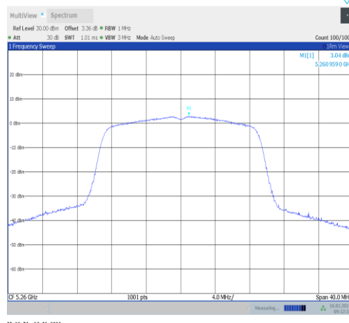
11n20ISO-Ant1-5260-PASS
