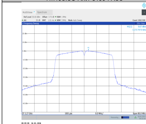
11n40SISO-Ant1-5270-PASS
