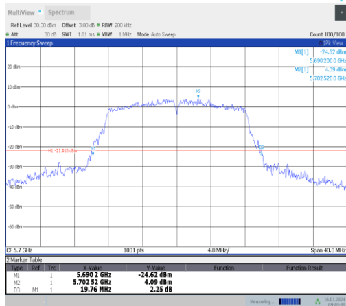
11a-Ant1-5700
