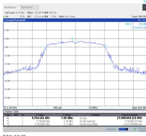
11a-Ant1-5745
