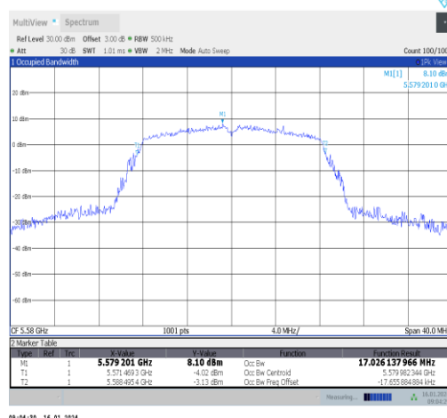
11a-Ant1-5580
