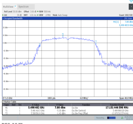
11a-Ant1-5500
