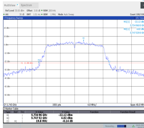
11a-Ant1-5745
