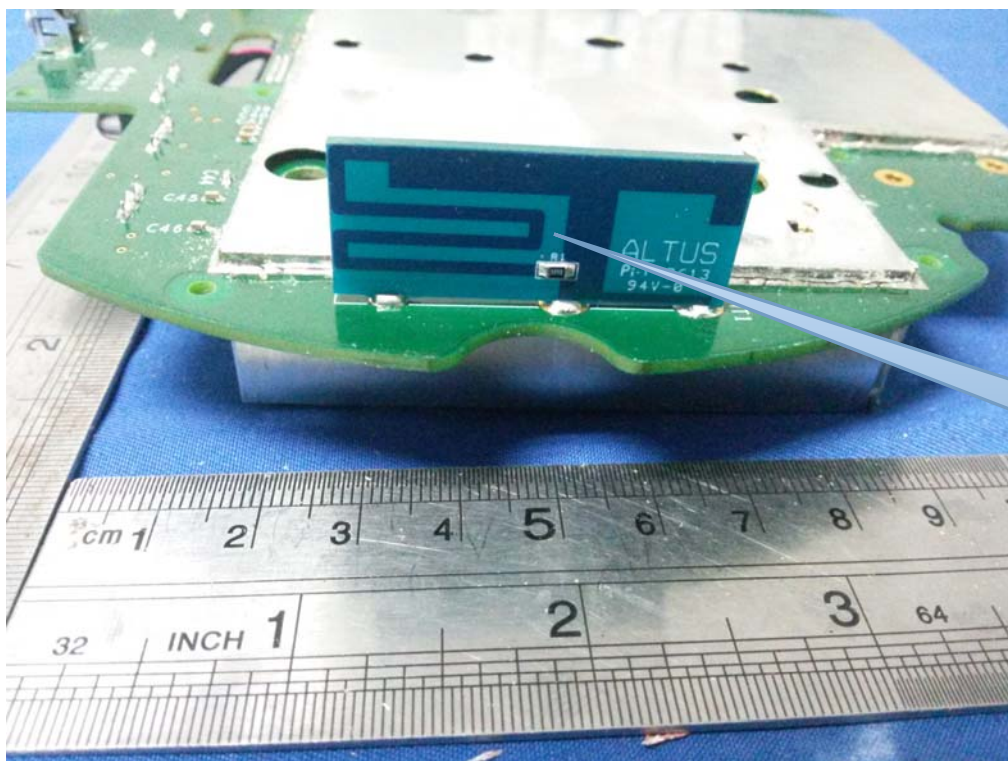
GSM antenna
