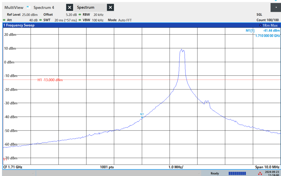
Band4-20MHz-QPSK-20050-6RB#0
