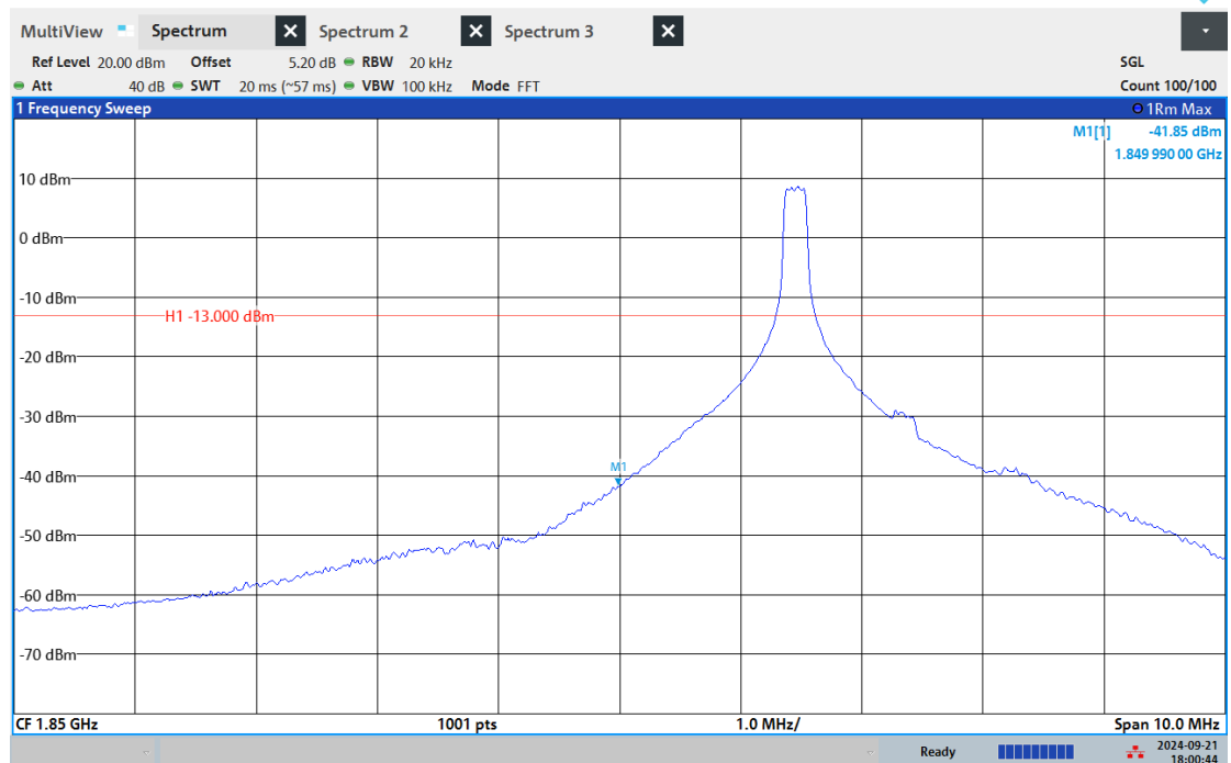
Band2-20MHz-16QAM-18700-6RB#0
