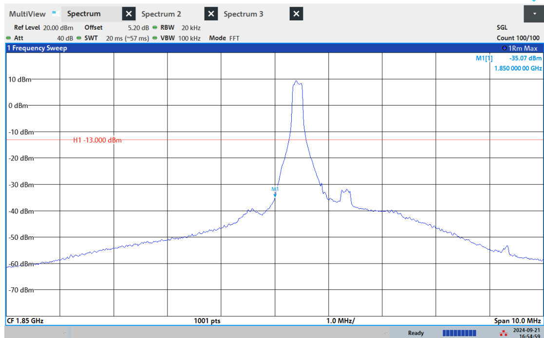
Band2-3MHz-QPSK-18615-6RB#0
