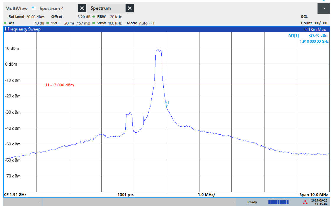
Band2-3MHz-QPSK-19185-6RB#0
