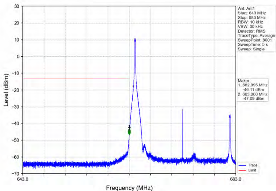
Band71_20MHz_16QAM_LCH_673MHz_RB_1_0_NTNV
