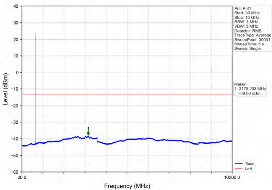
Band71_5MHz_QPSK_HCH_695.5MHz_RB_1_24_NTNV
