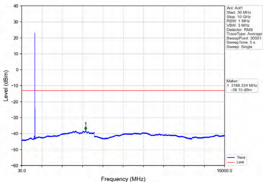
Band71_10MHz_QPSK_MCH_680.5MHz_RB_1_0_NTNV
