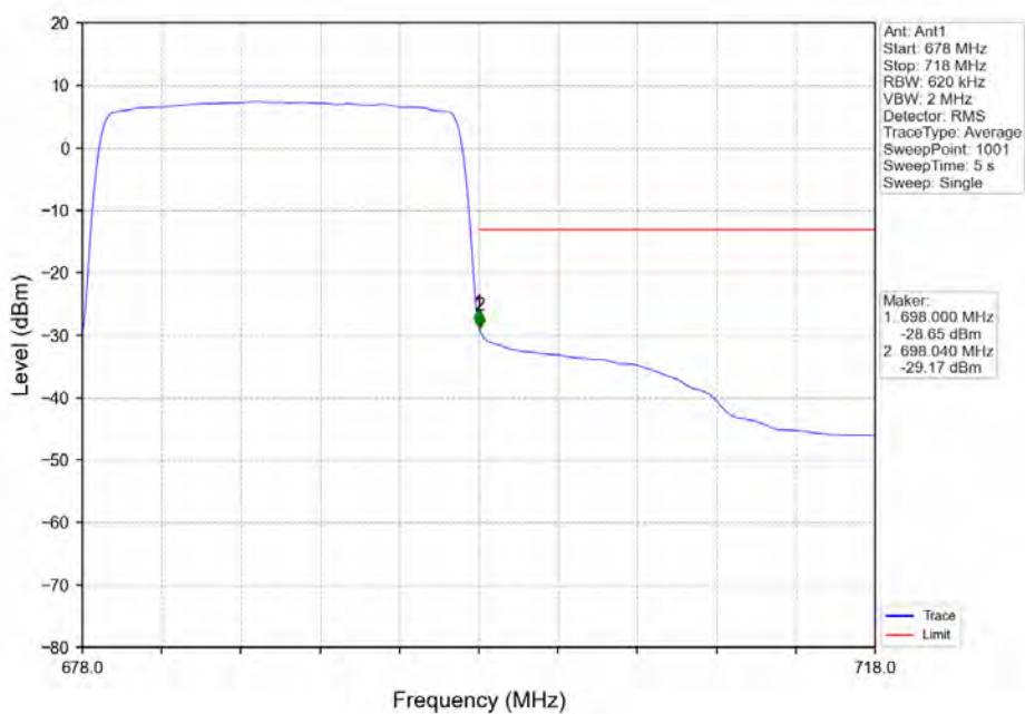
Band71_20MHz_16QAM_HCH_688MHz_RB_100_0_NTNV
