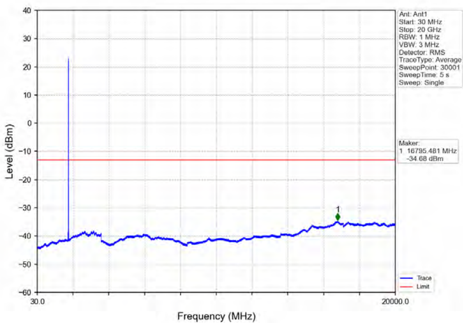
Band66_10MHz_QPSK_HCH_1775MHz_RB_1_49_NTNV
