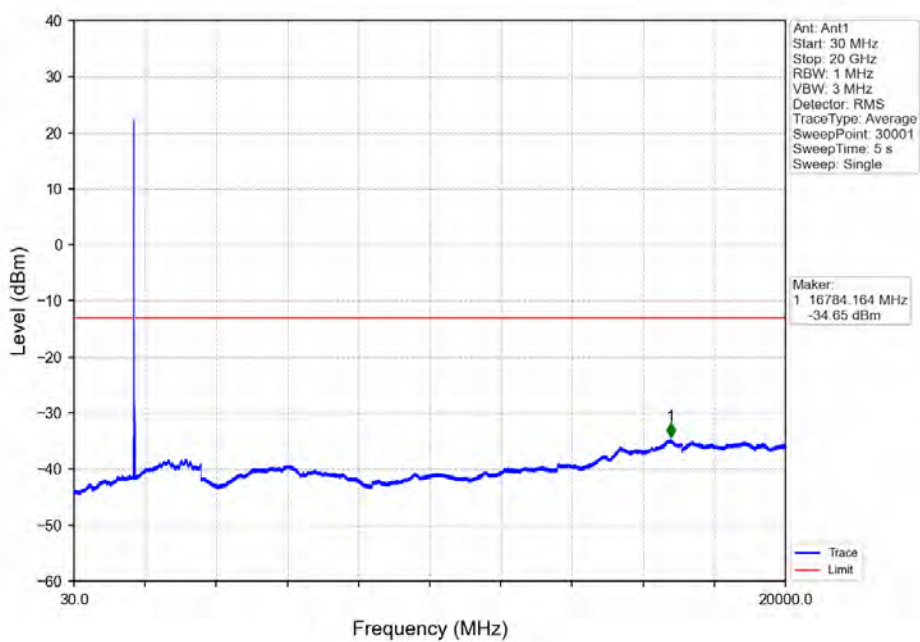
Band66_20MHz_16QAM_LCH_1720MHz_RB_100_0_NTNV
