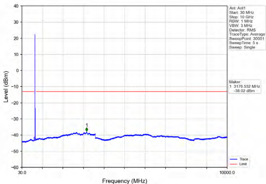
Band71_20MHz_16QAM_LCH_673MHz_RB_100_0_NTNV
