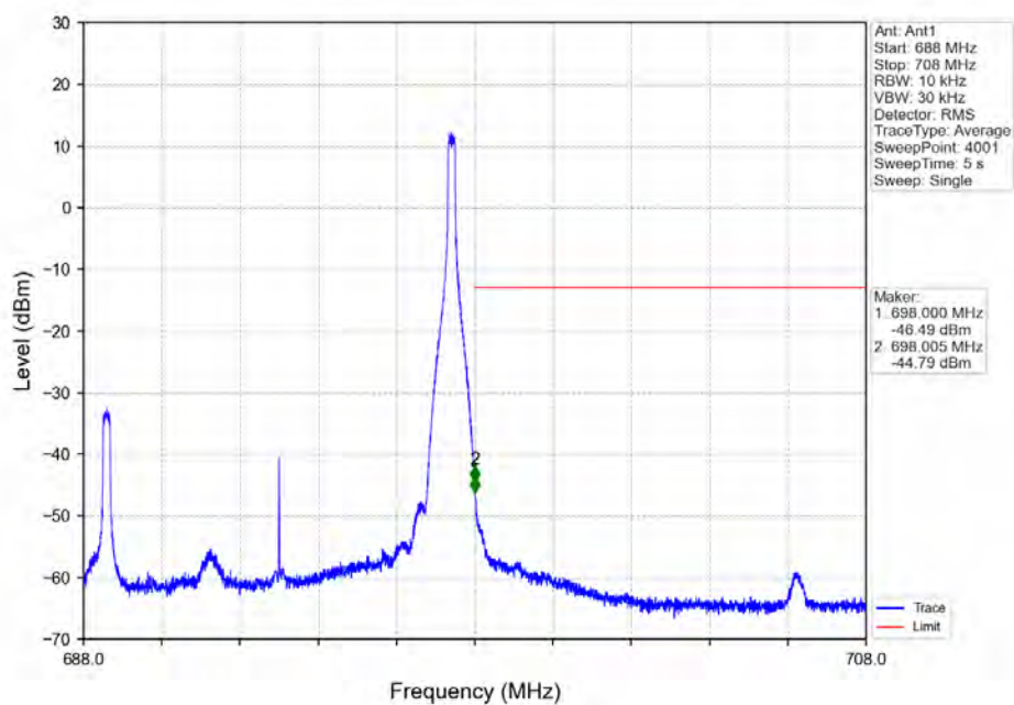
Band71_10MHz_QPSK_HCH_693MHz_RB_1_49_NTNV
