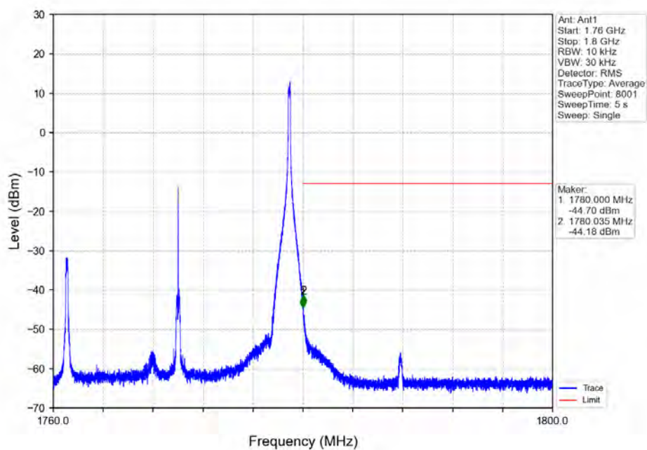
Band66_20MHz_QPSK_HCH_1770MHz_RB_1_99_NTNV
