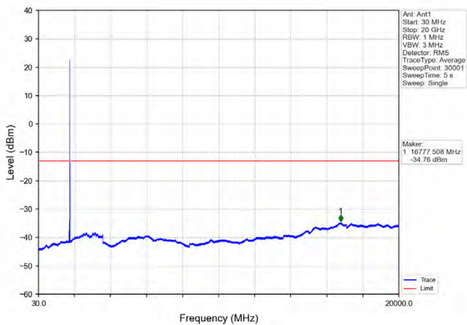
Band66_20MHz_QPSK_HCH_1770MHz_RB_1_99_NTNV
