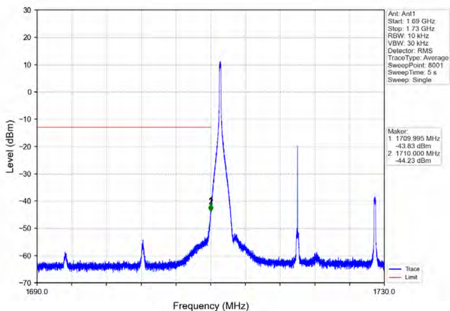
Band66_20MHz_16QAM_LCH_1720MHz_RB_1_0_NTNV
