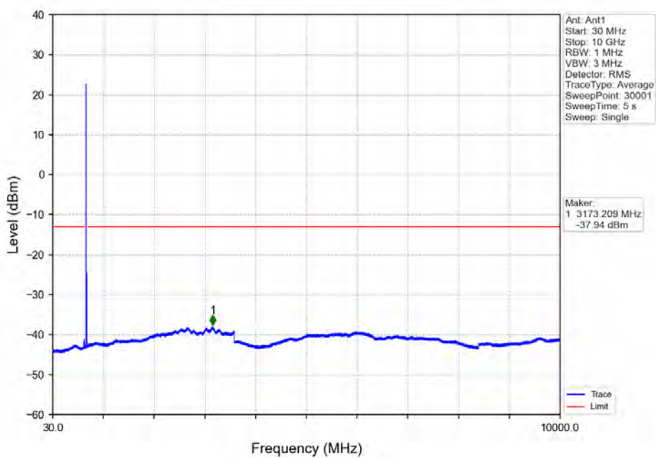
Band71_15MHz_QPSK_HCH_690.5MHz_RB_1_74_NTNV
