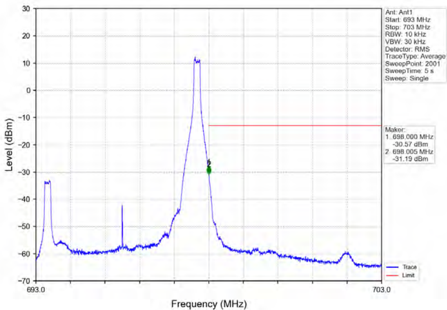
Band71_5MHz_QPSK_HCH_695.5MHz_RB_1_24_NTNV
