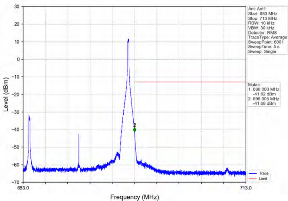
Band71_15MHz_QPSK_HCH_690.5MHz_RB_1_74_NTNV
