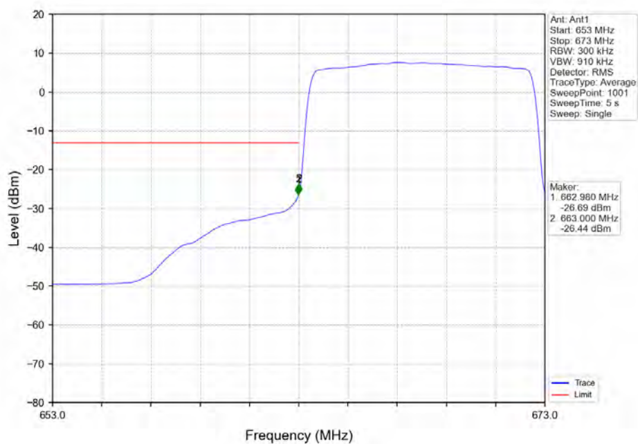
Band71_10MHz_16QAM_LCH_668MHz_RB_50_0_NTNV
