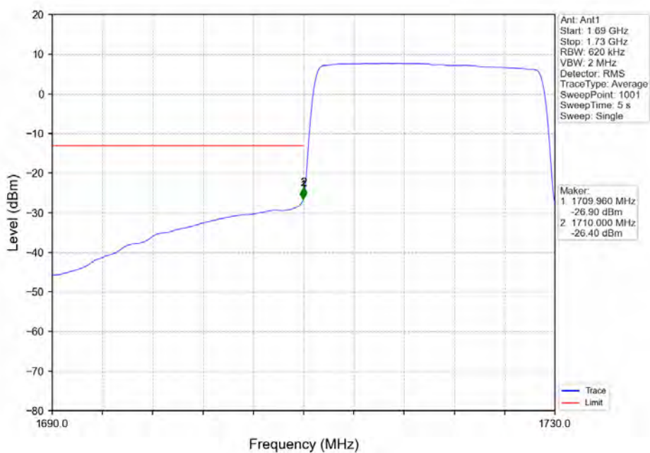
Band66_20MHz_16QAM_LCH_1720MHz_RB_100_0_NTNV
