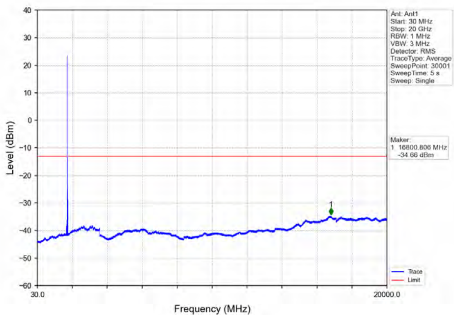
Band66_20MHz_QPSK_MCH_1745MHz_RB_1_0_NTNV
