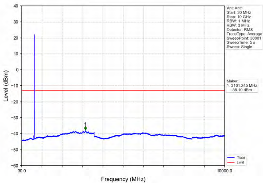
Band71_10MHz_16QAM_LCH_668MHz_RB_50_0_NTNV
