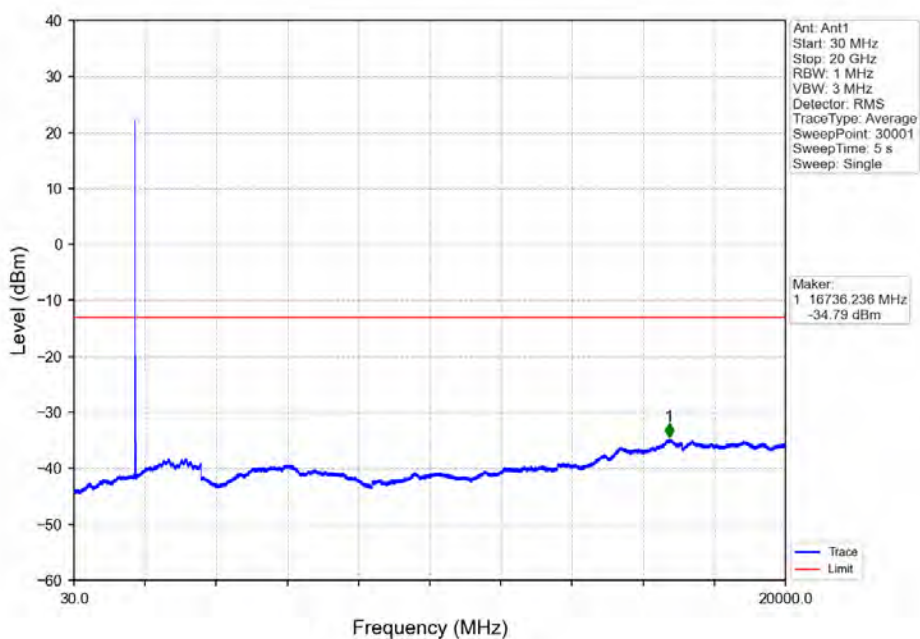
Band4_15MHz_QPSK_HCH_1747.5MHz_RB_1_74_NTNV
