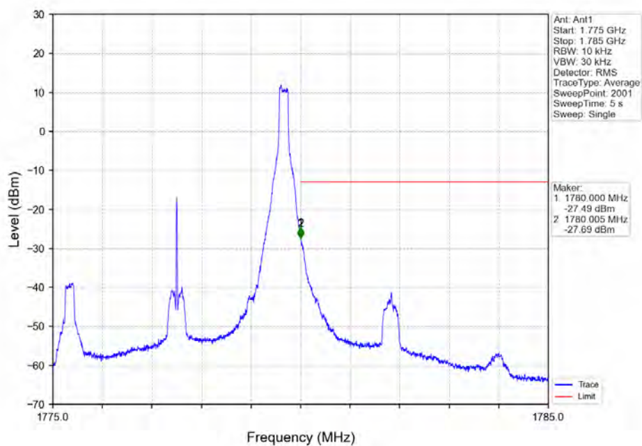
Band66_5MHz_QPSK_HCH_1777.5MHz_RB_1_24_NTNV
