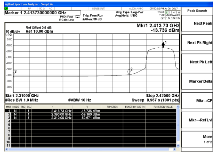
802.11n-HT20 Low channel(Average)
