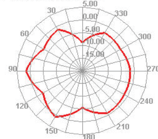
2500.000MHz E1
