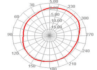
2400.000MHz E2
