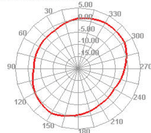
2450.000MHz H
