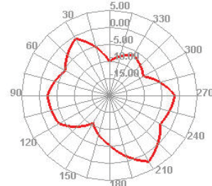
2450.000MHz E2
