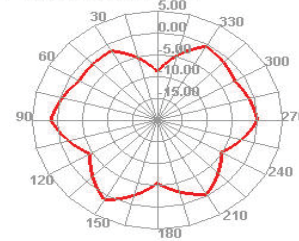
2400.000MHz E1
