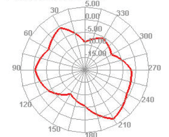
2500.000MHz E2
