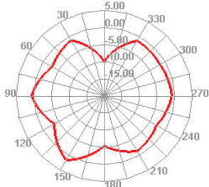
2450.000MHz E1
