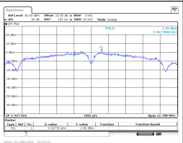
SISO Ant. 3
