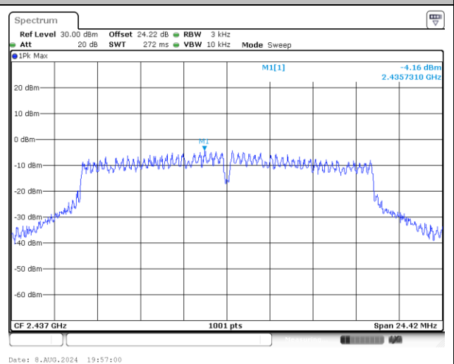
MIMO Ant 3
