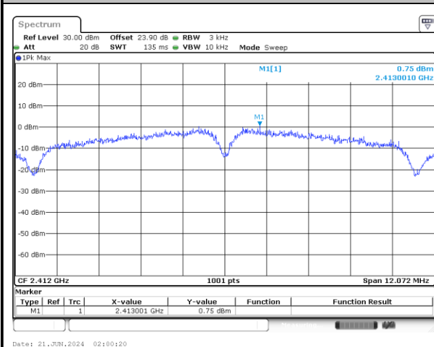
SISO Ant. 4
