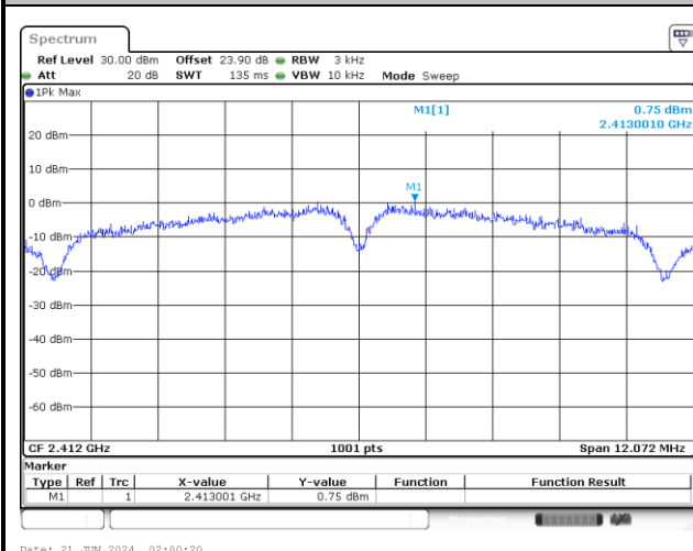
SISO Ant. 4
