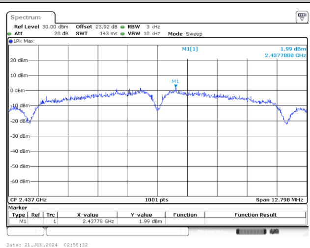
SISO Ant. 3
