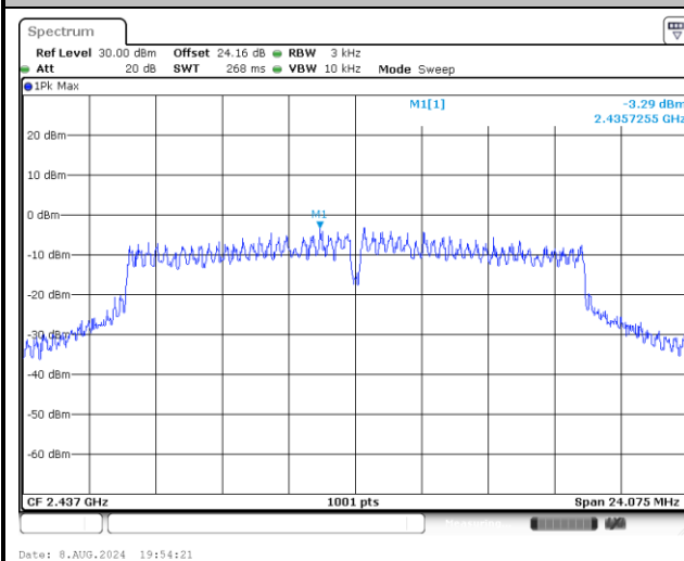
MIMO Ant 4
