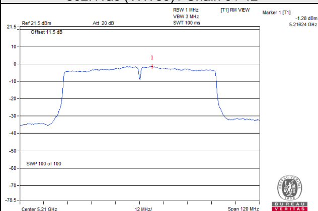
802.11ac (VHT80) / Chain 0 / 42
