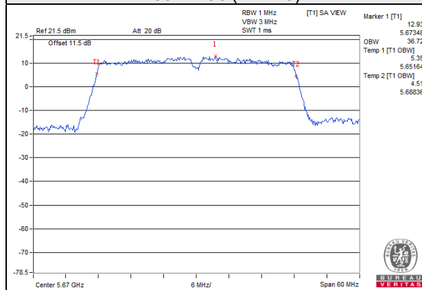
802.11ac (VHT40)
