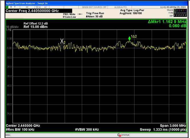
8DPSK
