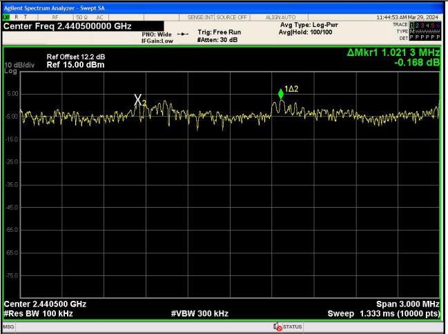
8DPSK
