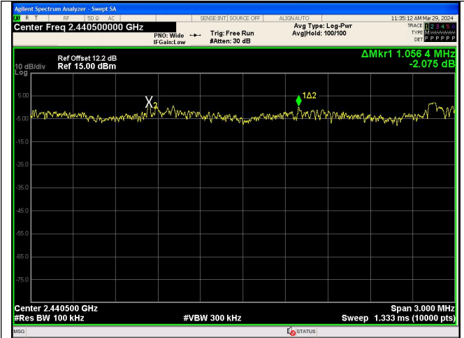
\pi/4 DQPSK
