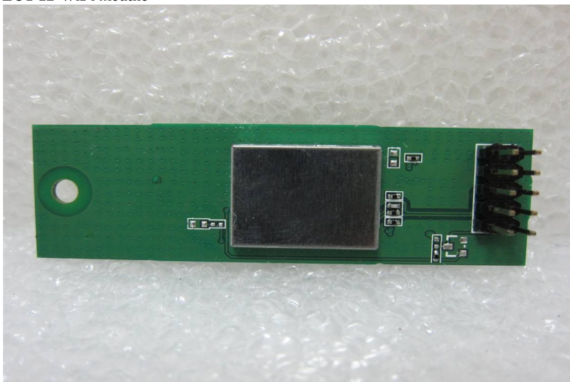
EUT 12 WiFi module
