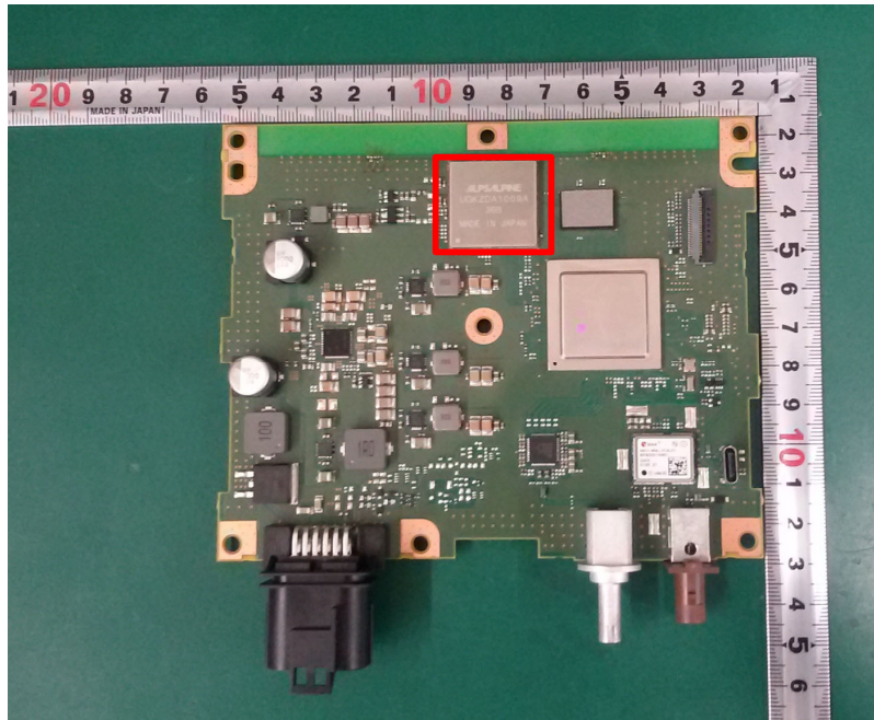
BT/WiFi Module
