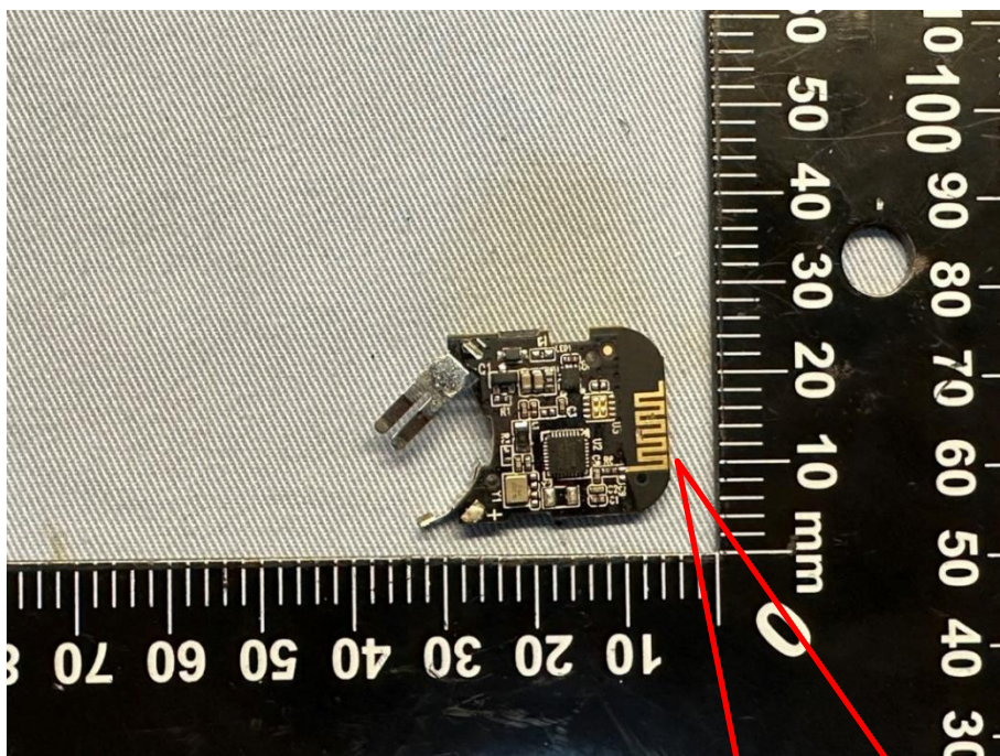
06. Antenna
