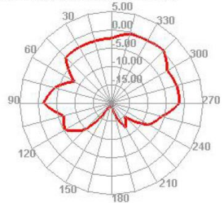
2500.000MHz Phi=45
