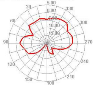
2450.000MHz Phi=45
