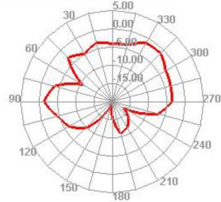
2400.000MHz Phi=45
