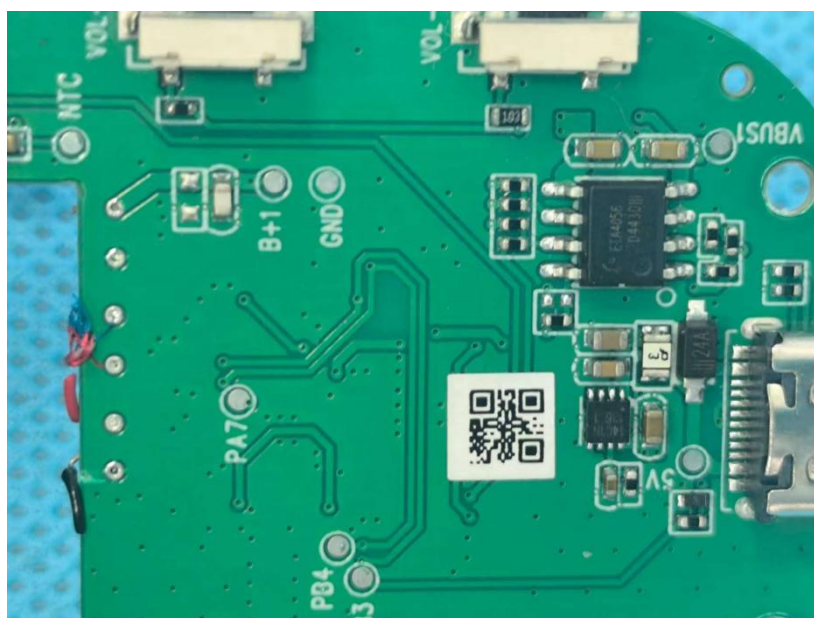
EUT Photo
