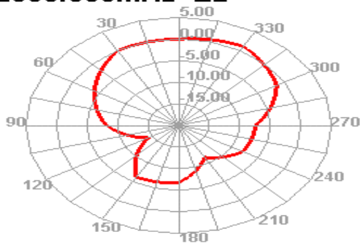
2500.000MHz E2
