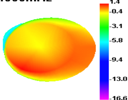
2500.000MHz
