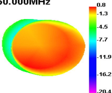
2450.000MHz E1
