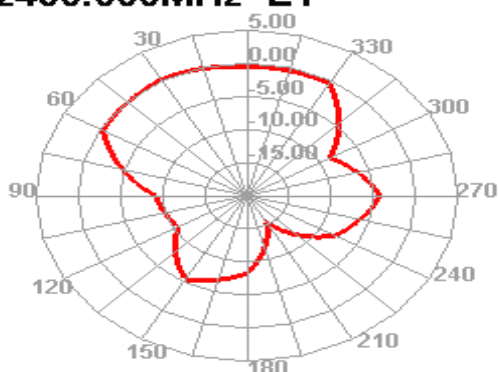
2450.000MHz E1
