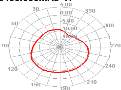
2450.000MHz H
