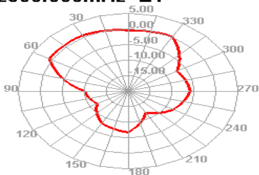
2500.000MHz E1
