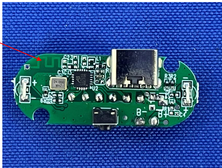
PCR Antenna
