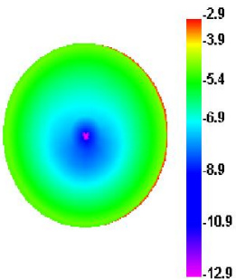
440.000MHz
