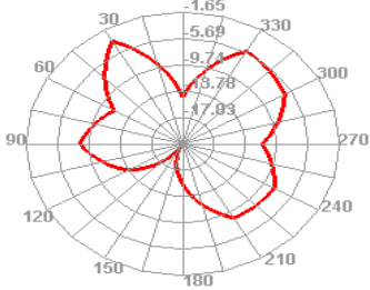
5400.000MHz E1
