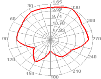
5400.000MHz E2
