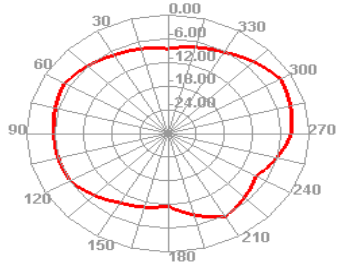
5400.000MHz H
