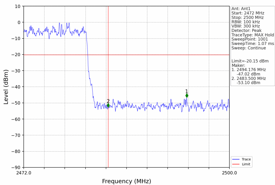
Pi/4DQPSK_2DH5_HOPP_Ant1_NTNV
