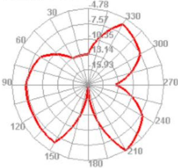
433.000MHz E2
