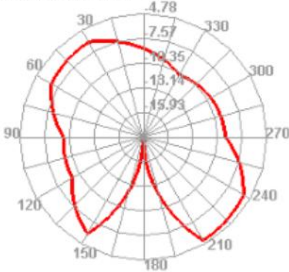
433.000MHz E1
