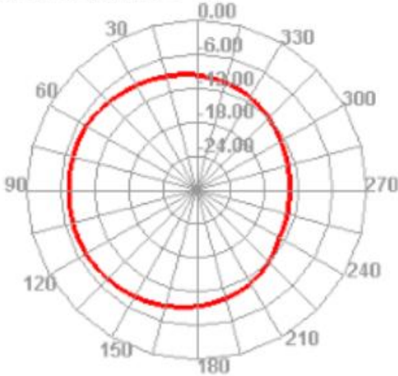
433.000MHz H
